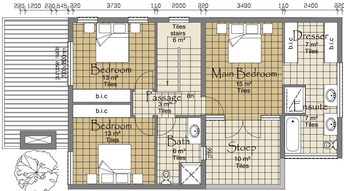
1:100 Unit A3 & A5 - First Floor Plan
